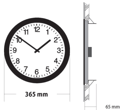
Außendurchmesser Einbau H x T: 350 +5 mm
